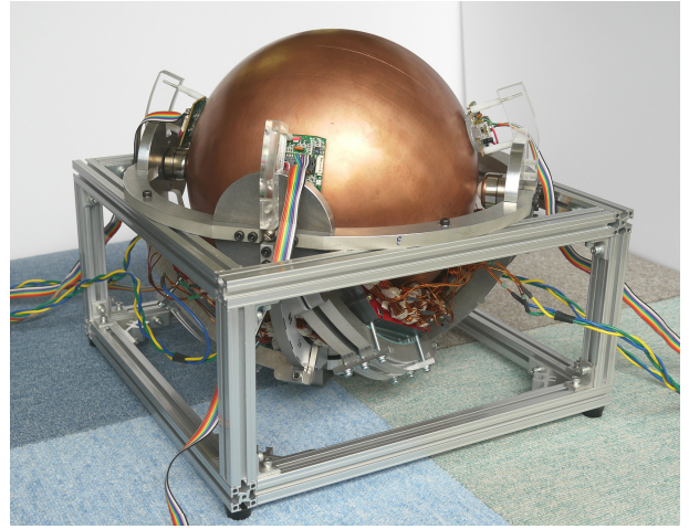
球面誘導モータ試作機の外観
