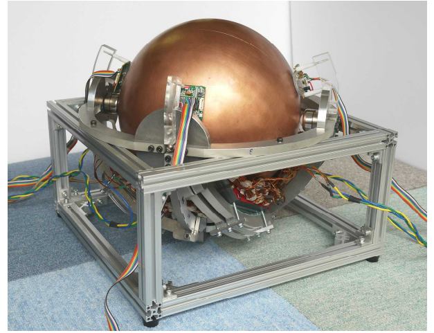
球面誘導モータ試作機の外観
