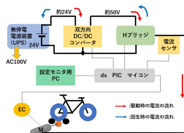
システムブロック図
