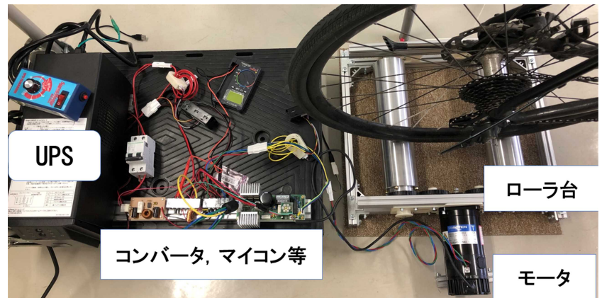
実験システム全体図
