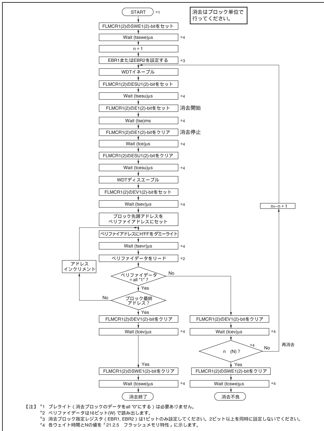
図 18.12 イレース/イレースペリファイロー（単一ブロック消去）
