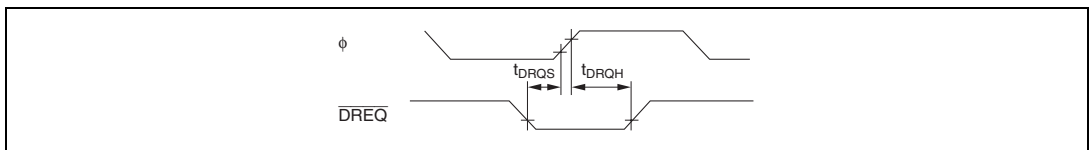
図 21.26 DMAC \overline{DREQ} 入力タイミング
