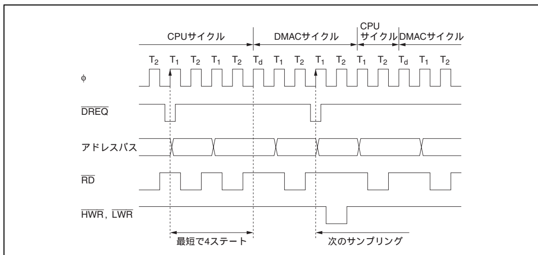
図 8.16 ノーマルモード時の \overline{DREQ} 端子の立ち下がりエッジによる DMAC 起動タイミング
