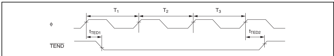
図 21.25 DMAC \overline{TEND} 出力タイミング / 3 ステートアクセス
