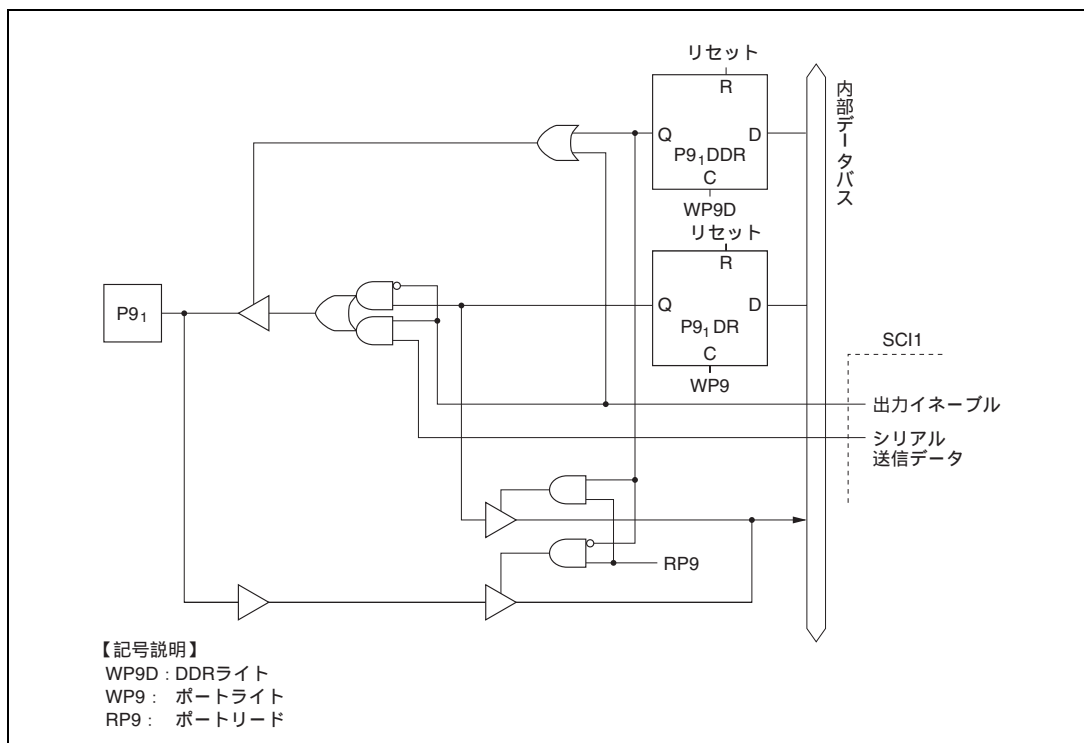
図 C.9 (b) ポート9 ブロック図 (P9 1 端子)
