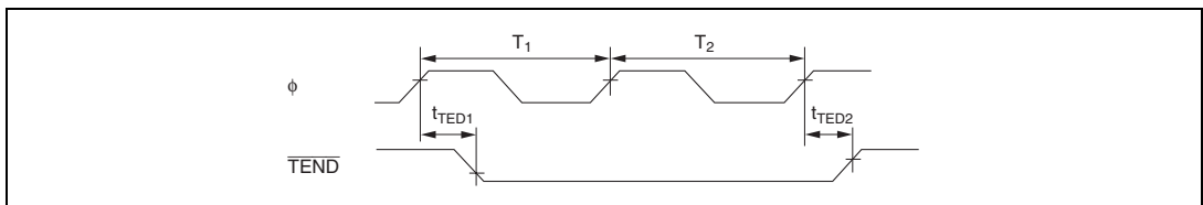
図 21.24 DMAC \overline{TEND} 出力タイミング / 2 ステートアクセス
