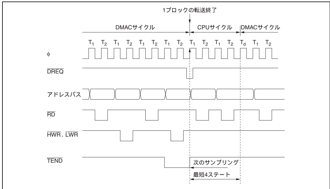
図 8.18 ブロック転送モード時の \overline{DREQ} 端子の立ち下がりエッジによる DMAC 起動タイミング
